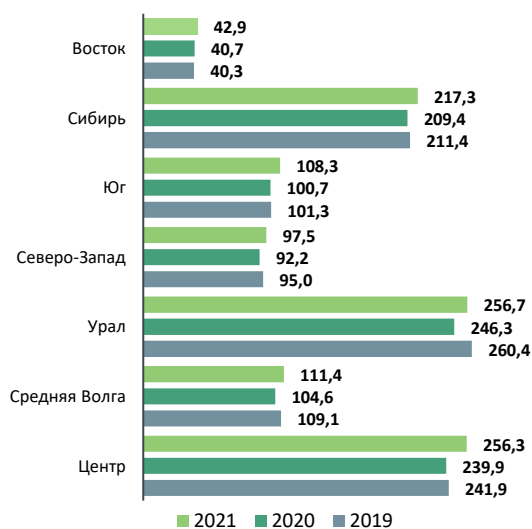
Рисунок 4. Потребление по ОЭС за год, млрд кВт*ч
